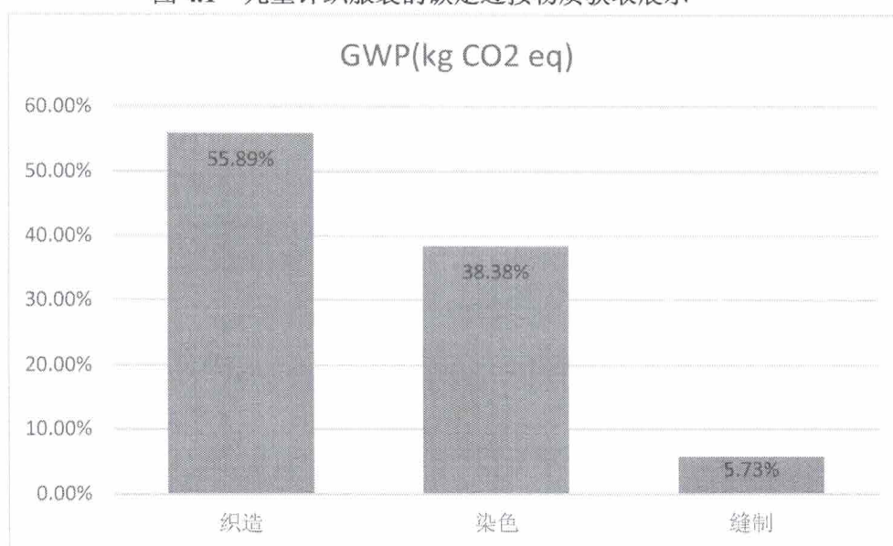
图 4.2 儿童针织服装的碳足迹按过程展示
